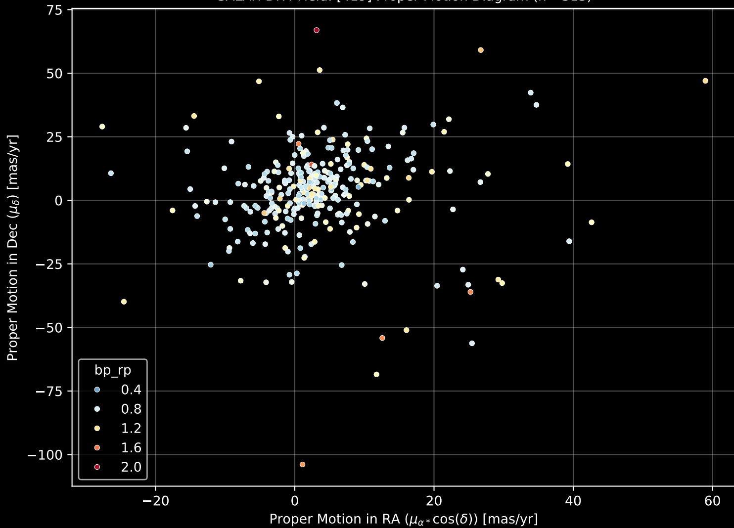
GALAH DR4 Field: [419] Proper Motion Diagram (n= 313)
