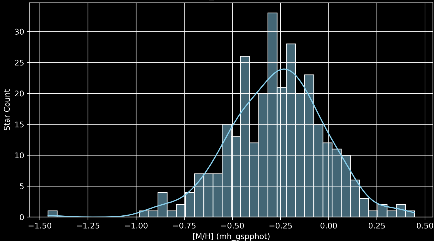
GALAH DR4 Field: [419] [M/H] (mh_gspphot) (n= 310)
