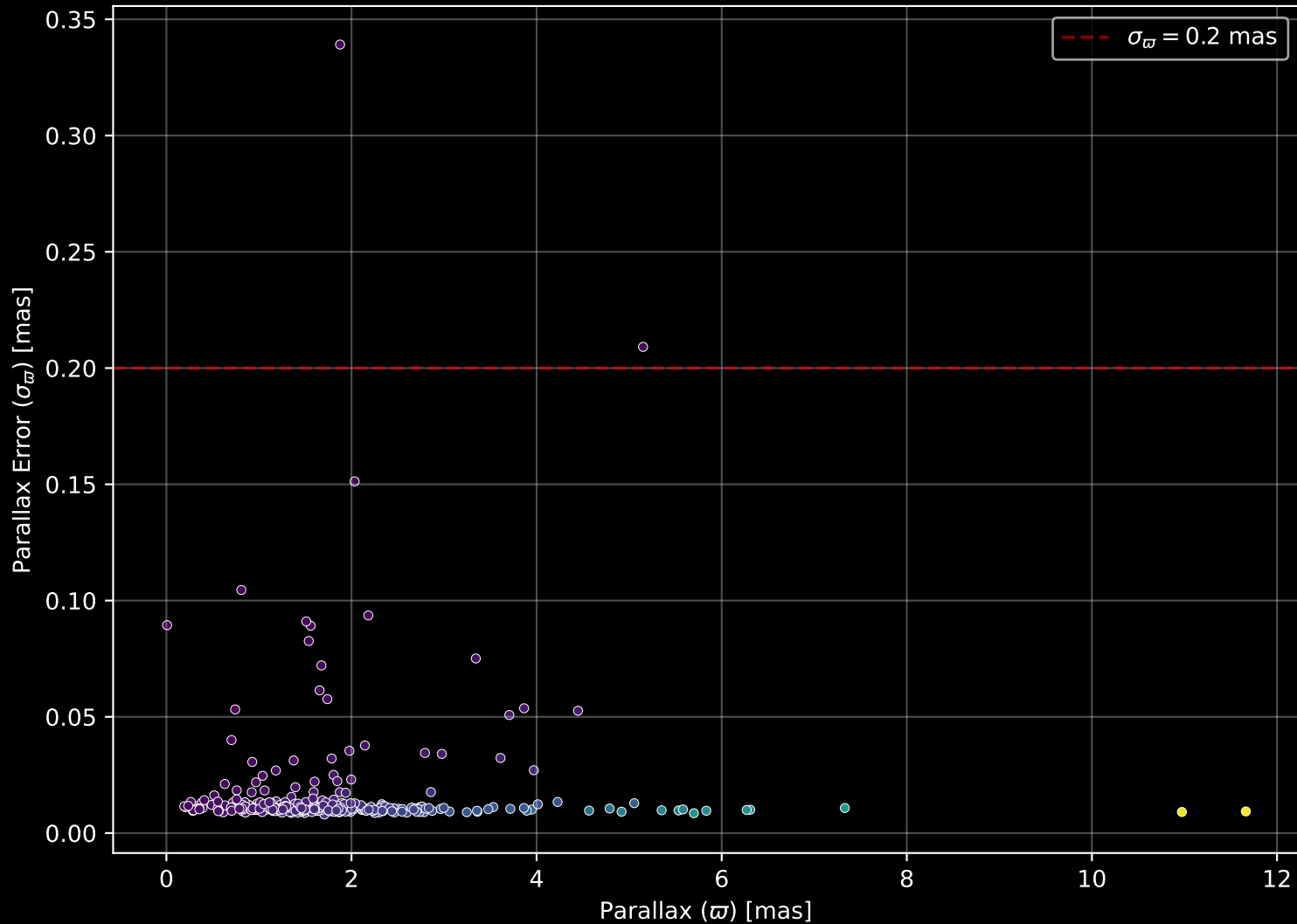
GALAH DR4 Field: [419] Parallax Quality (n= 313)
