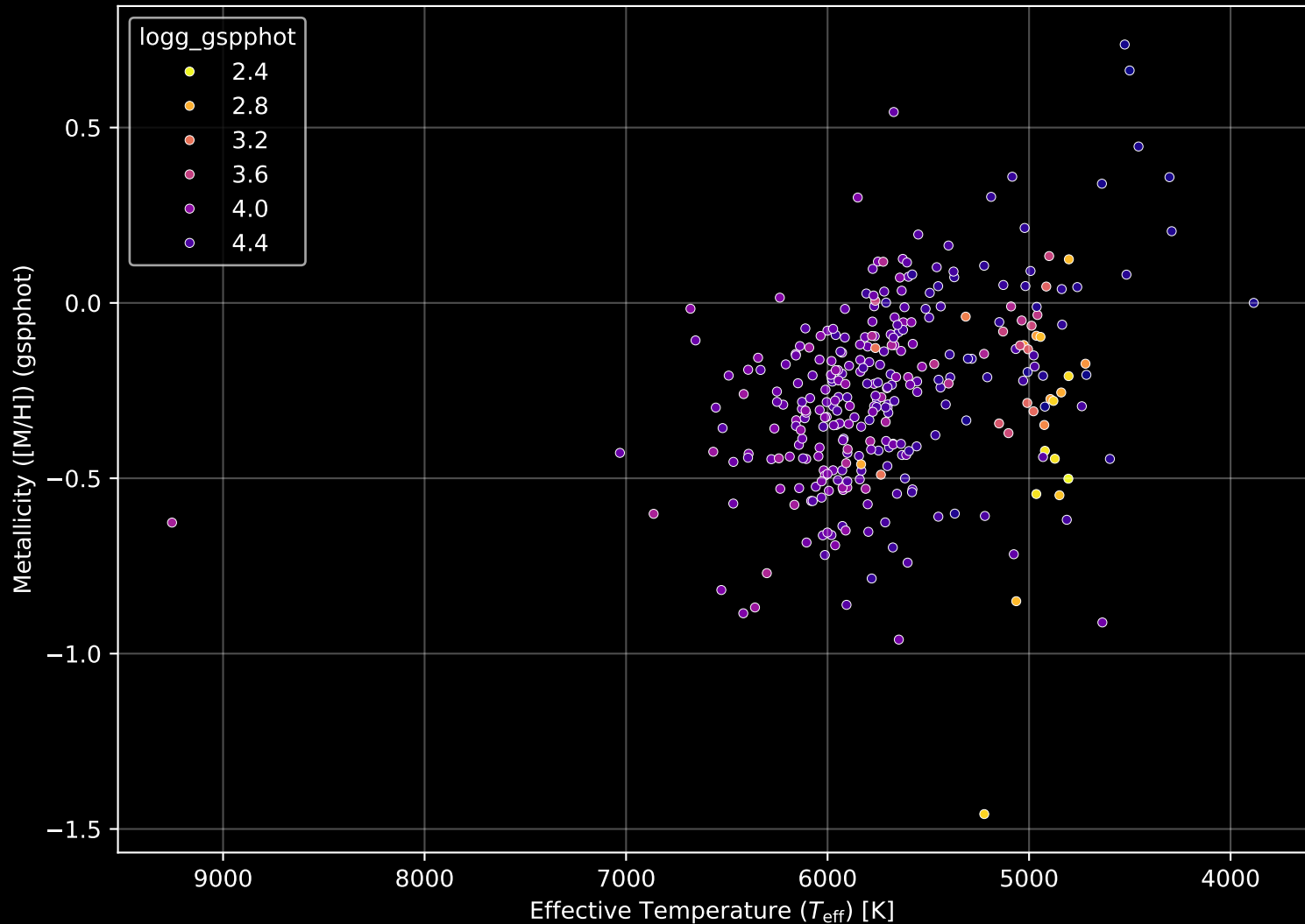
GALAH DR4 Field: [419] Stellar Population Parameters (n= 313)
